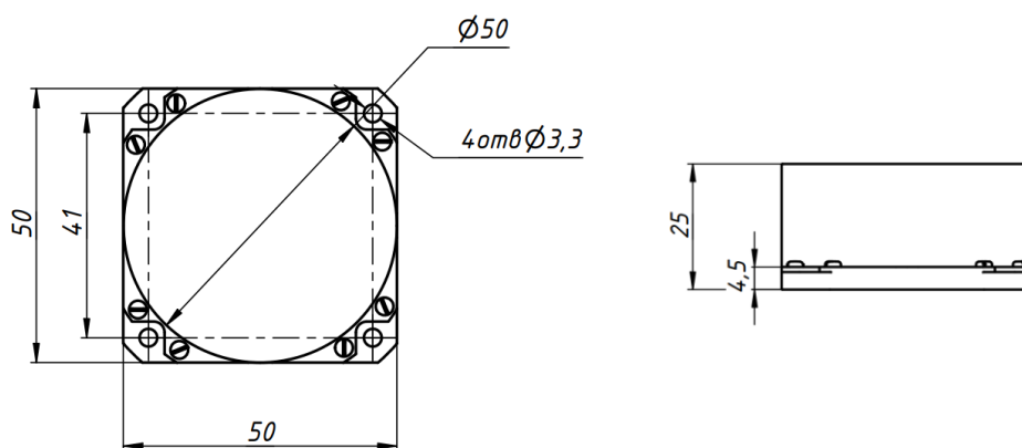
Рисунок 1. Габаритные размеры
